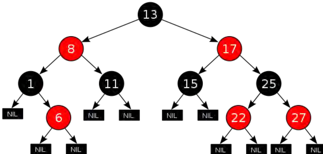
Figura 42: Ejemplo de un árbol red-black.
