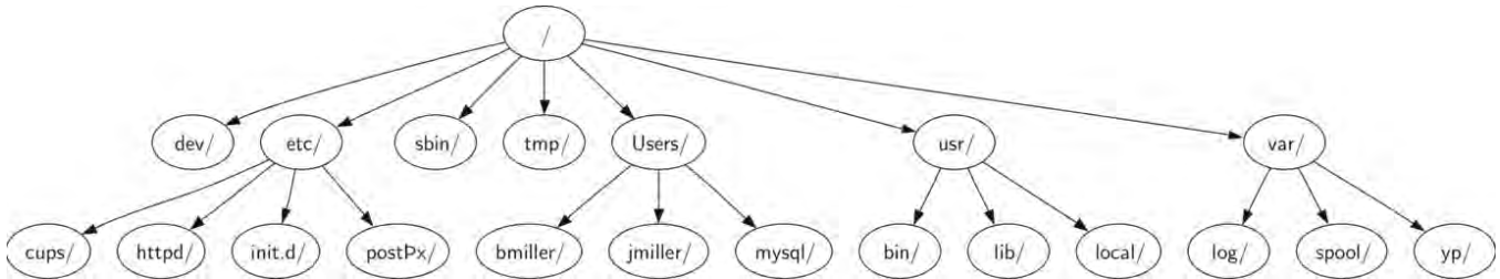
Figura 21: El árbol representa el sistema de archivos en Unix. En un sistema de archivos existen archivos y directorios como una estructura de árbol.
